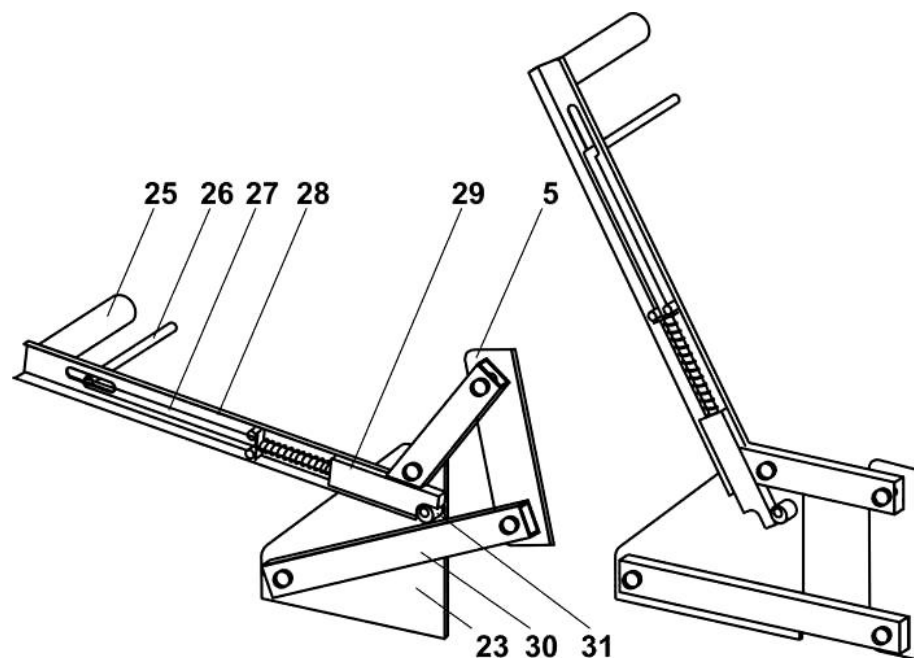
Рисунок 3. Подъемный механизм.
