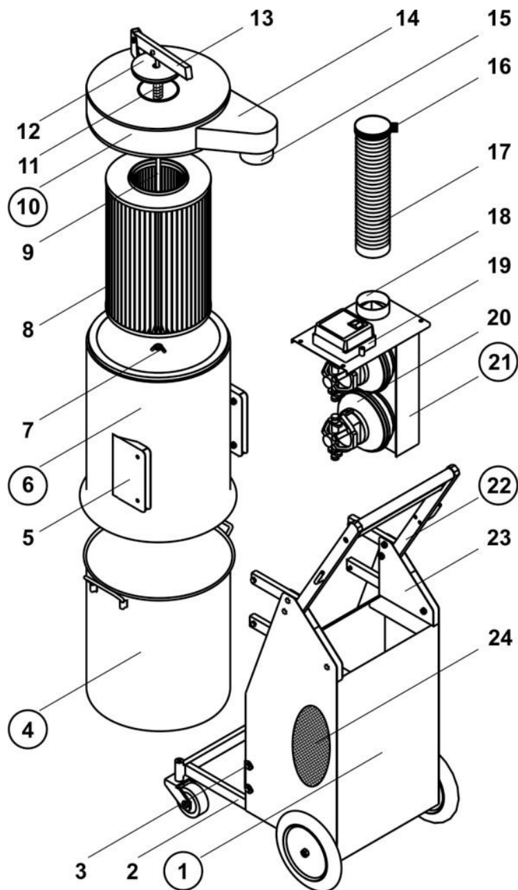
Рисунок 2. Устройство пылесоса.
