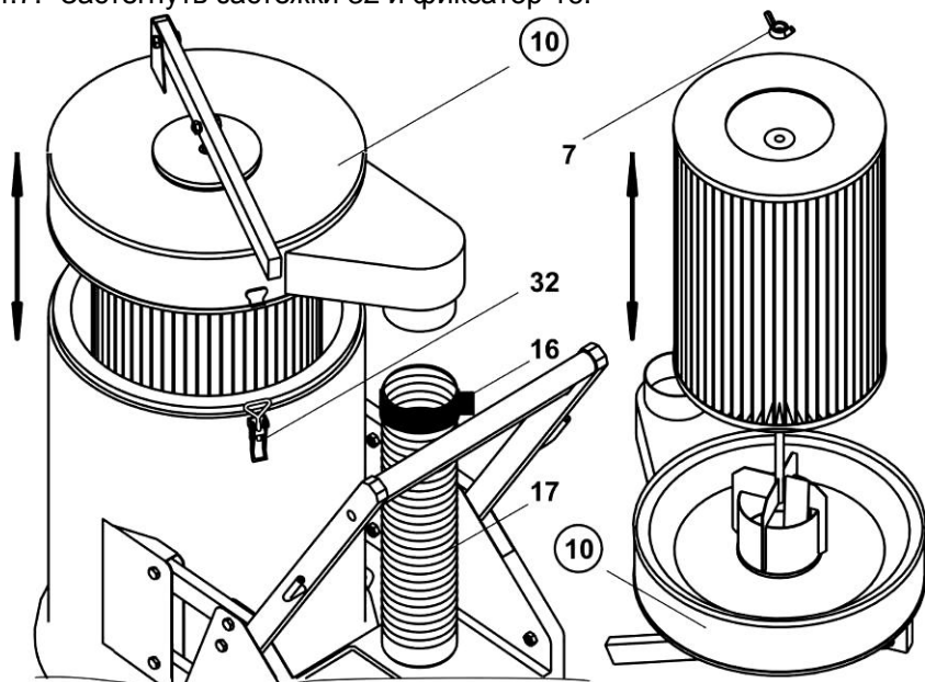
Рисунок 6. Замена фильтра.
